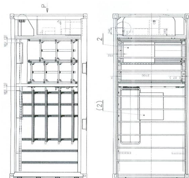
Mortuary Container - Interior Conteneur mortuaire - intérieur
